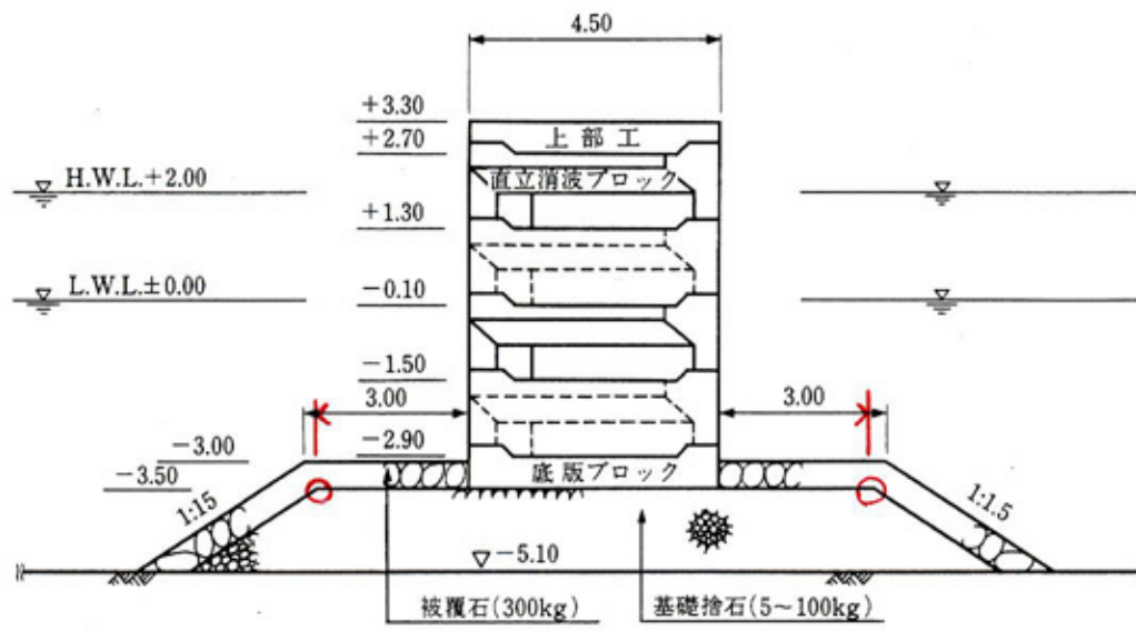
図2-6-9 標準断面図
